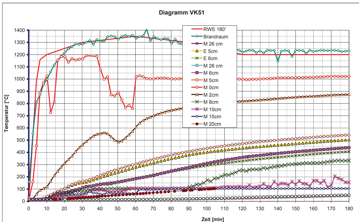
Abb. 37: Sondentemperaturen VK51
