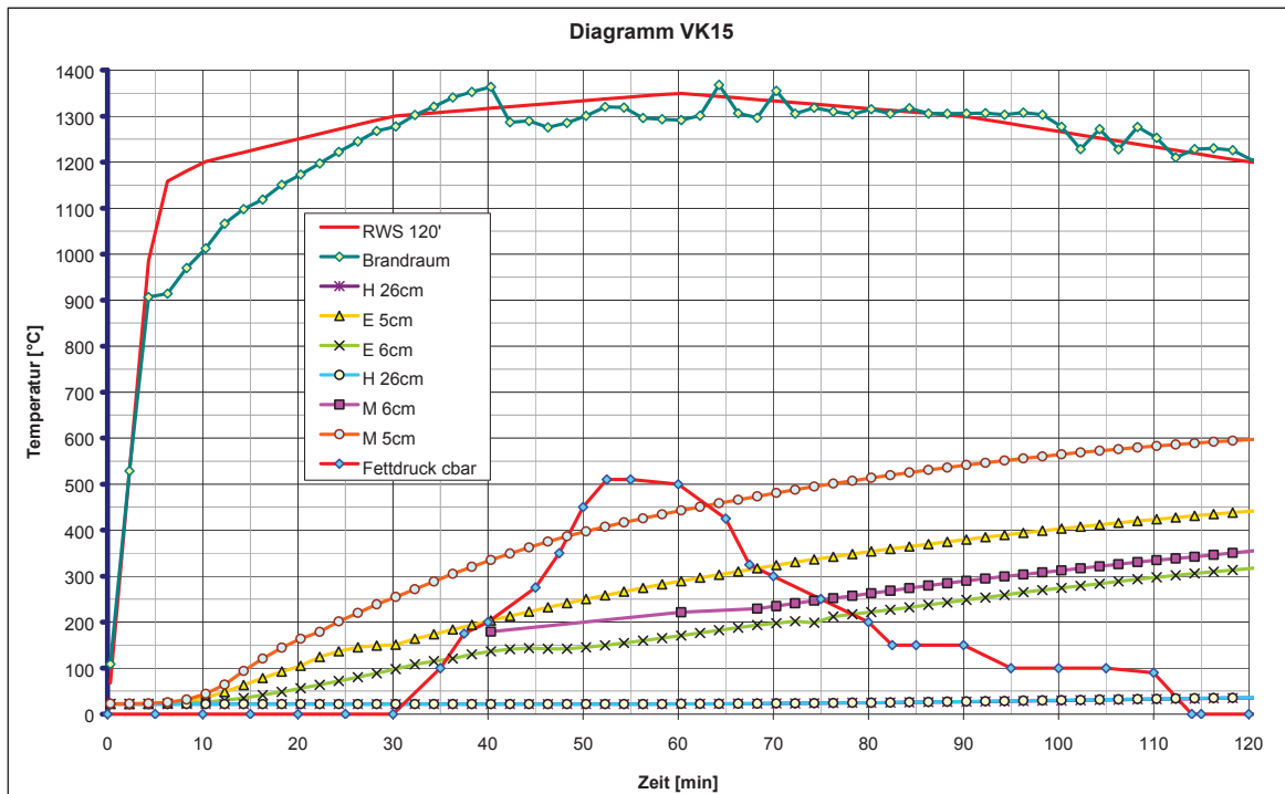
Abb. 15: Sondentemperaturen VK15
