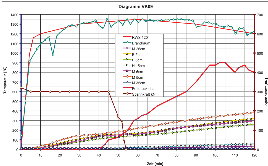
Abb. 9: Sondentemperaturen VK09
