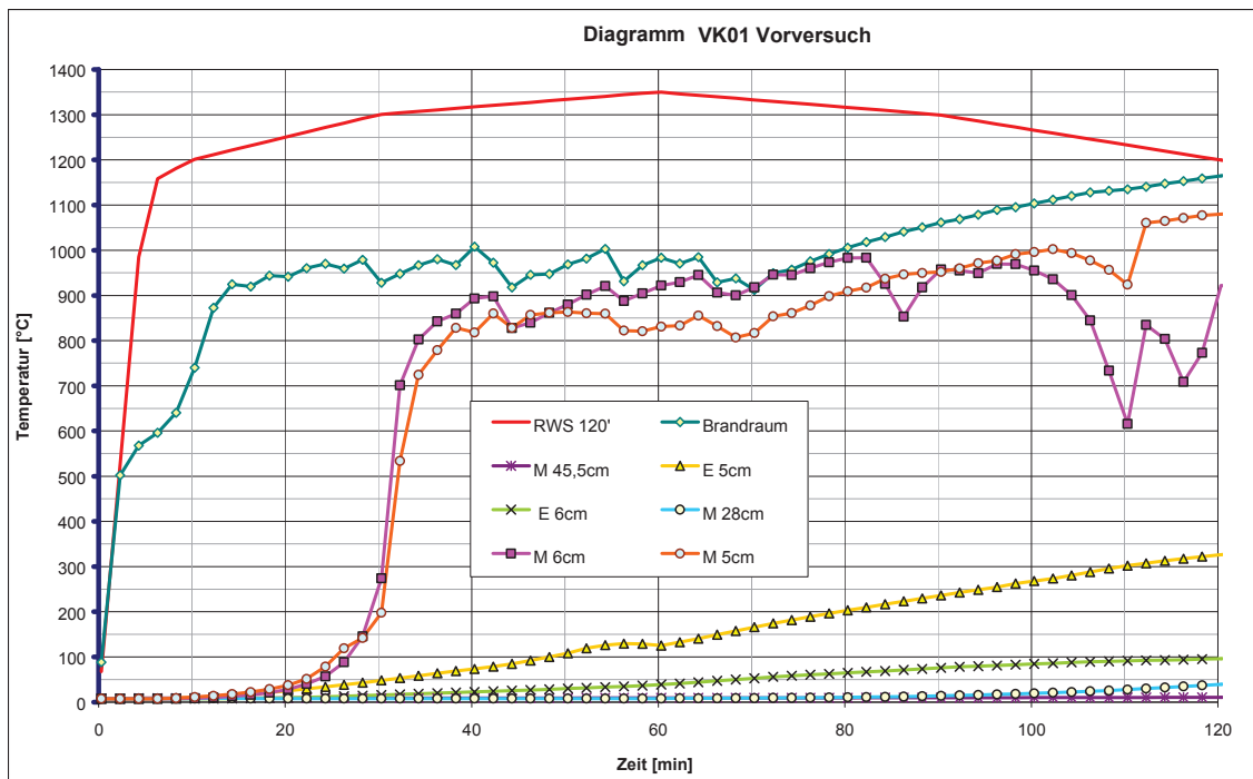
Abb. 1: Sondentemperaturen VK01
