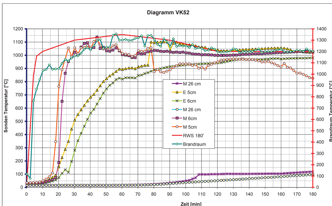
Abb. 38: Sondentemperaturen VK52
