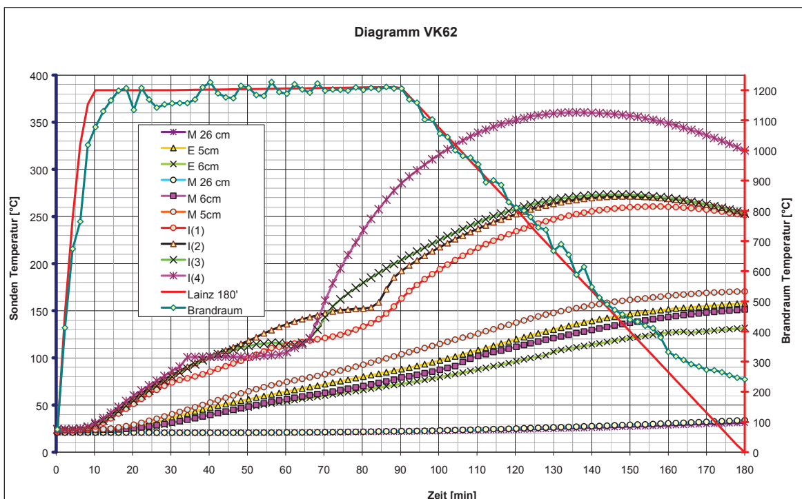
Abb. 44: Sondentemperaturen VK62
