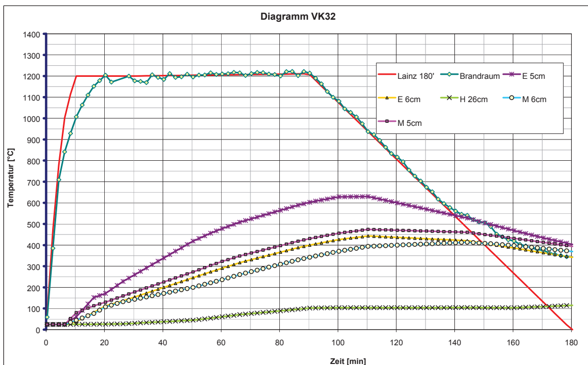
Abb. 30: Sondentemperaturen VK32
