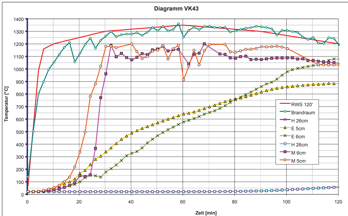
Abb. 35: Sondentemperaturen VK43
