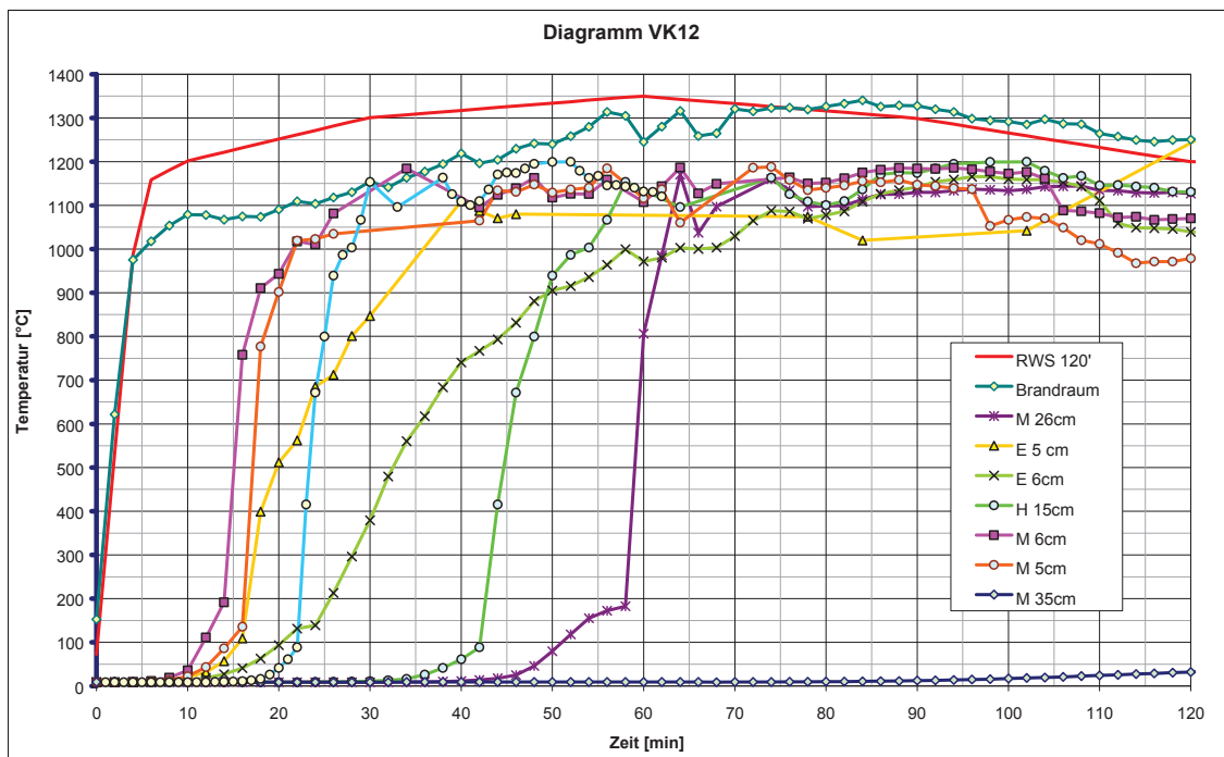
Abb. 12: Sondentemperaturen VK12
