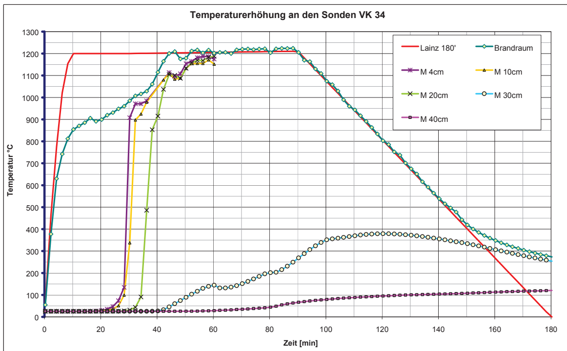
Abb. 32: Sondentemperaturen VK34
