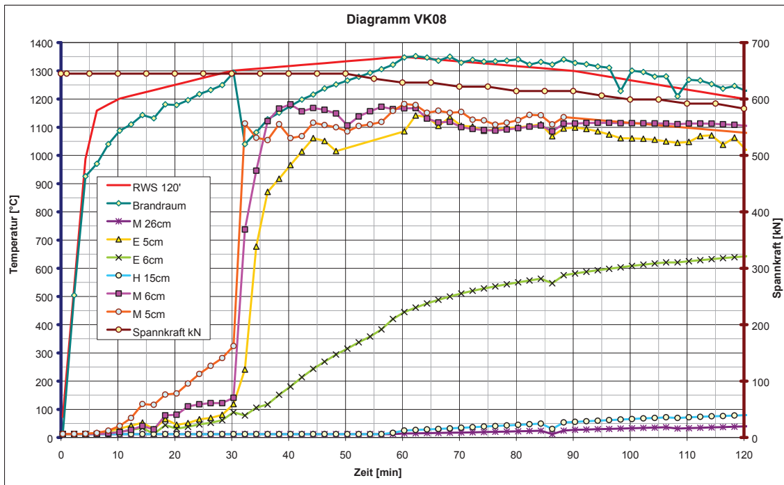
Abb. 8: Sondentemperaturen VK08
