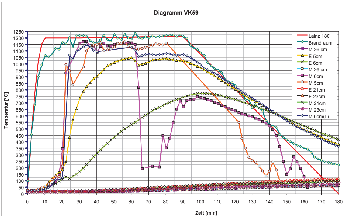
Abb. 42: Sondentemperaturen VK59
