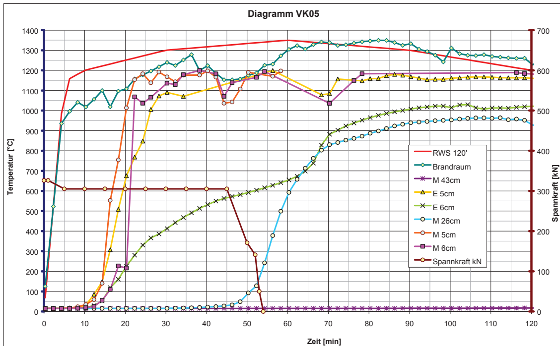
Abb. 5: Sondentemperaturen VK05
