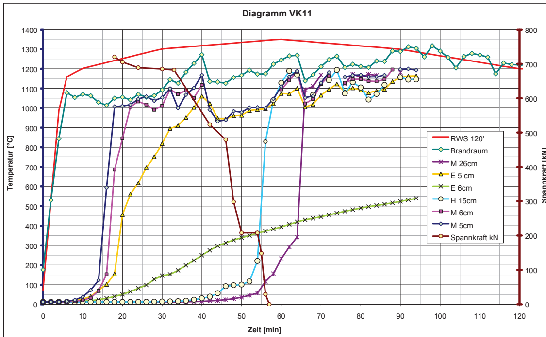
Abb. 11: Sondentemperaturen VK11
