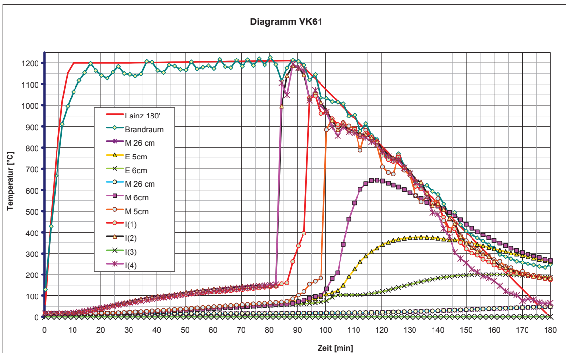
Abb. 43: Sondentemperaturen VK61
