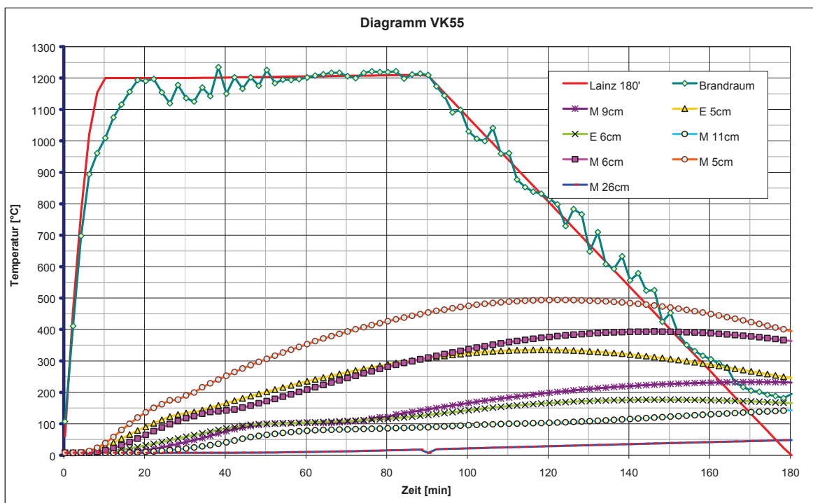
Abb. 40: Sondentemperaturen VK55
