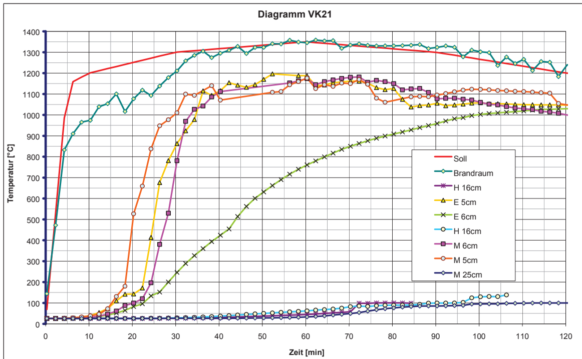
Abb. 21: Sondentemperaturen VK21
