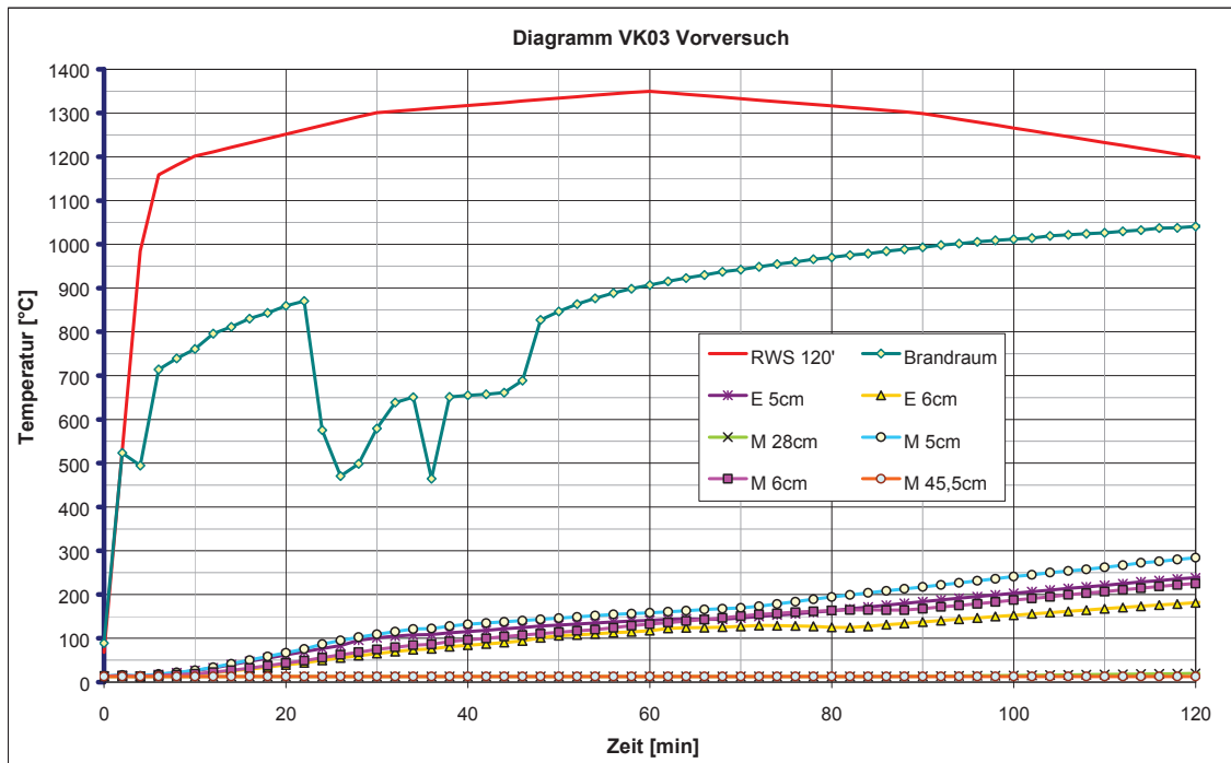
Abb. 3: Sondentemperaturen VK03
