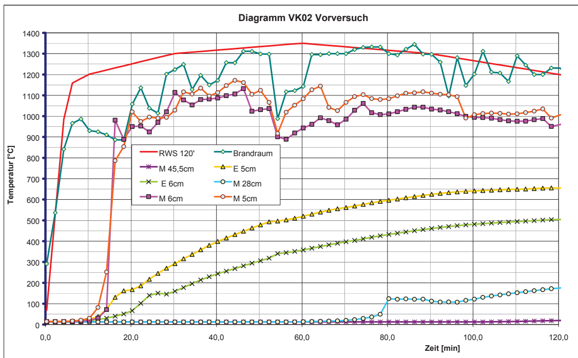
Abb. 2: Sondentemperaturen VK02
