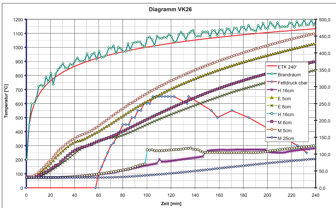
Abb. 26: Sondentemperaturen VK26 (doppelte Skalierung)
