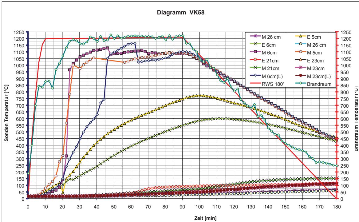
Abb. 41: Sondentemperaturen VK58
