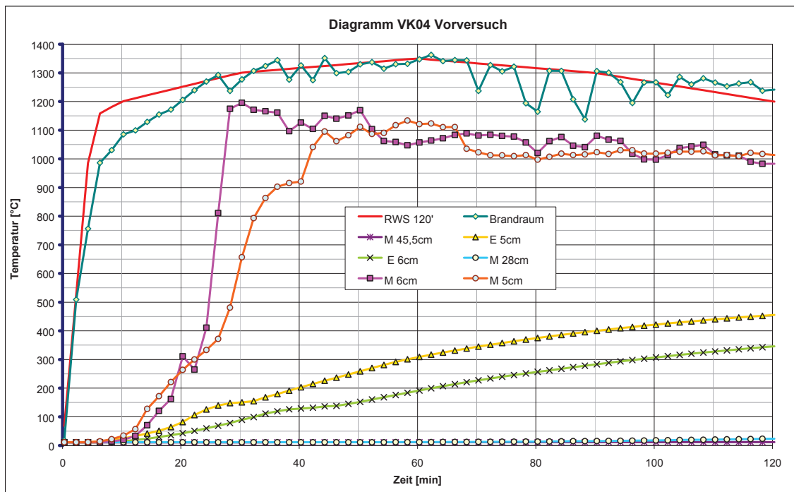
Abb. 4: Sondentemperaturen VK04
