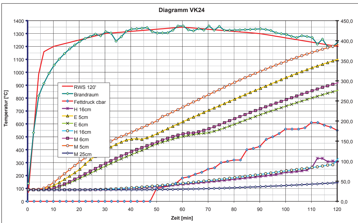
Abb. 24: Sondentemperaturen VK24 (doppelte Skalierung)
