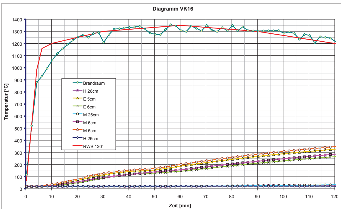
Abb. 16: Sondentemperaturen VK16
