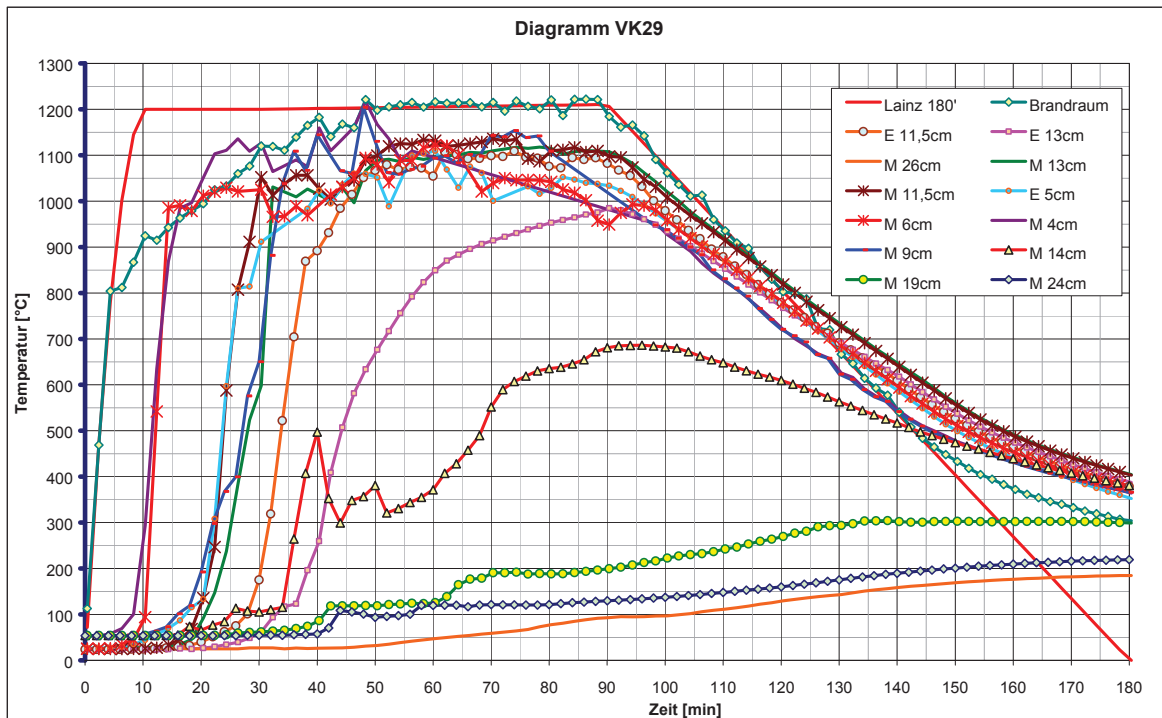
Abb. 27: Sondentemperaturen VK29
