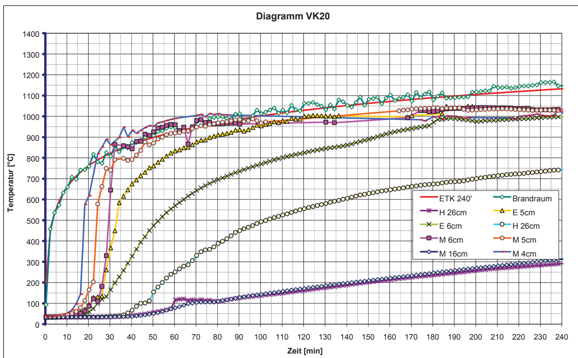
Abb. 20: Sondentemperaturen VK20
