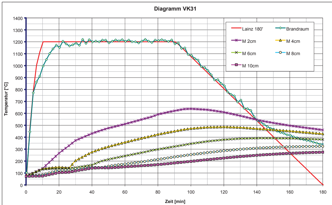
Abb. 29: Sondentemperaturen VK31
