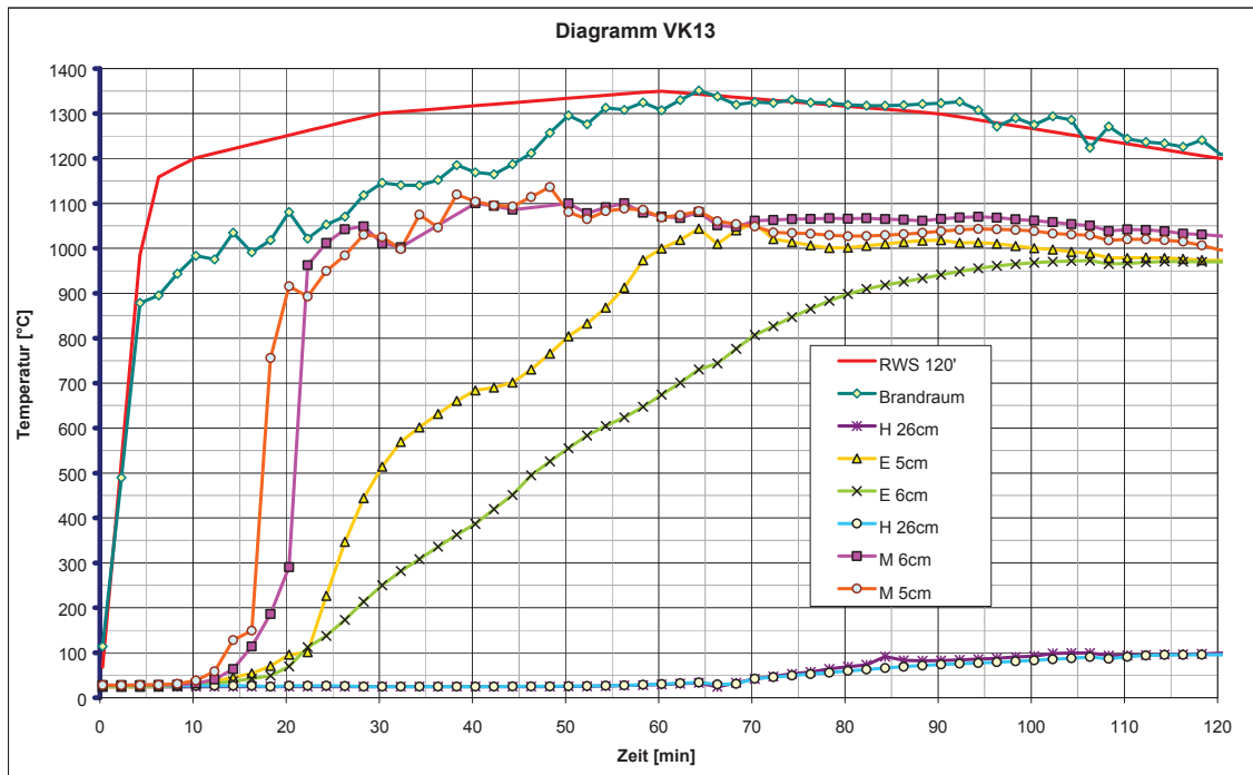
Abb. 13: Sondentemperaturen VK13
