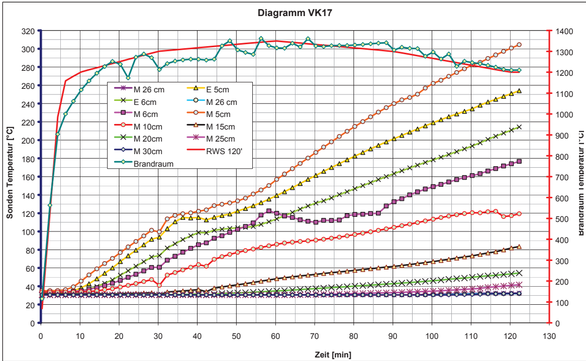
Abb. 17: Sondentemperaturen VK17 (doppelte Skalierung)
