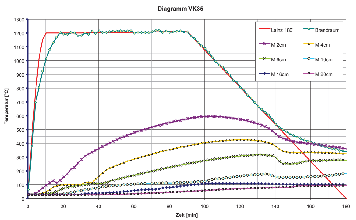
Abb. 33: Sondentemperaturen VK35
