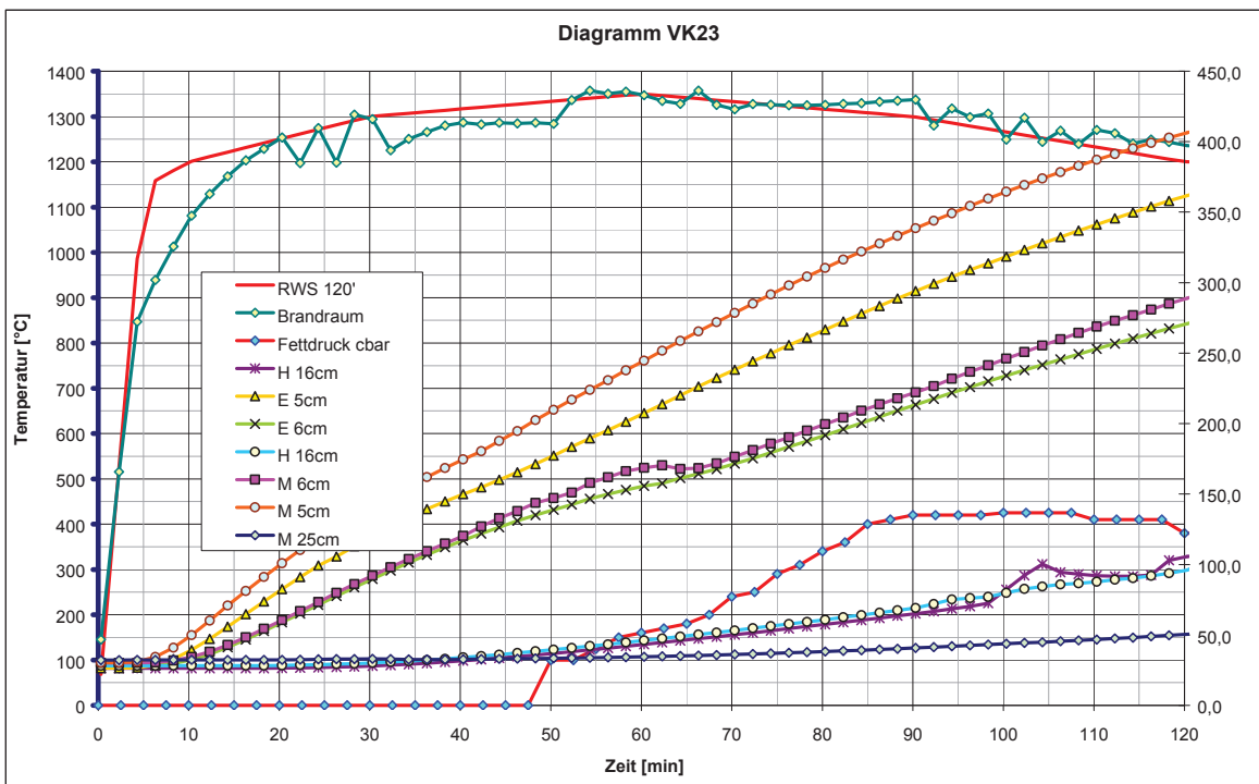
Abb. 23: Sondentemperaturen VK23 (doppelte Skalierung)
