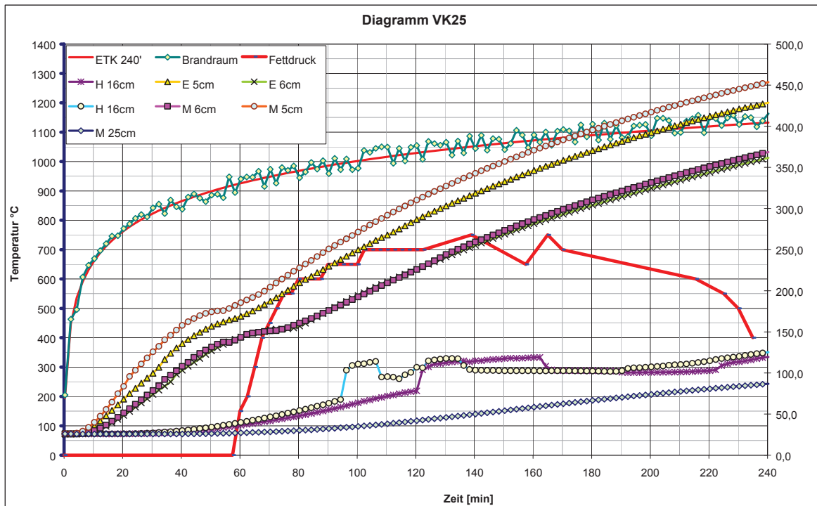
Abb. 25: Sondentemperaturen VK25 (doppelte Skalierung)
