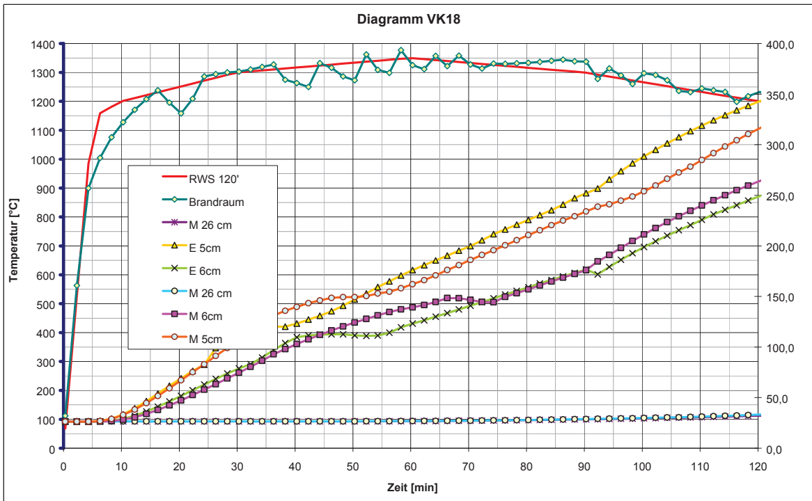
Abb. 18: Messwerte VK18 (doppelte Skalierung)
