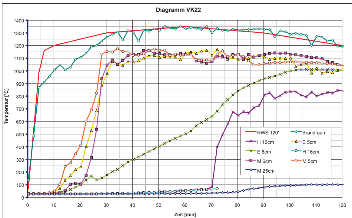
Abb. 22: Sondentemperaturen VK22
