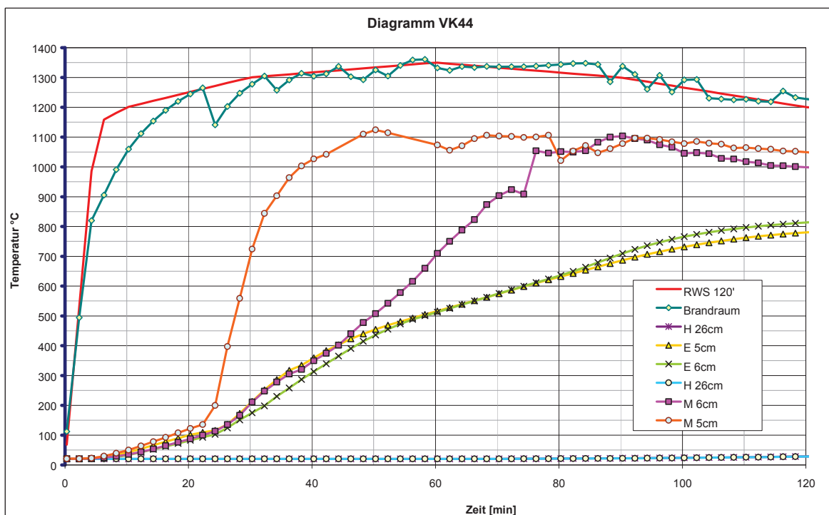
Abb. 36: Sondentemperaturen VK44
