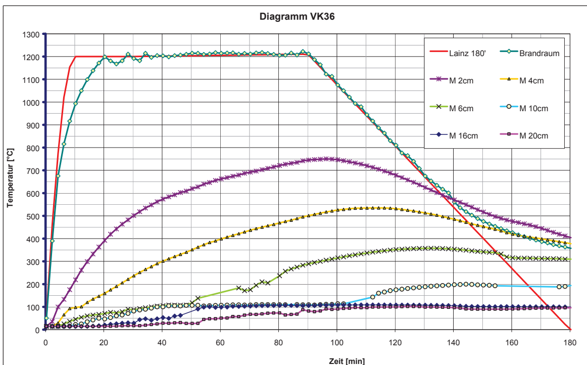
Abb. 34: Sondentemperaturen VK36
