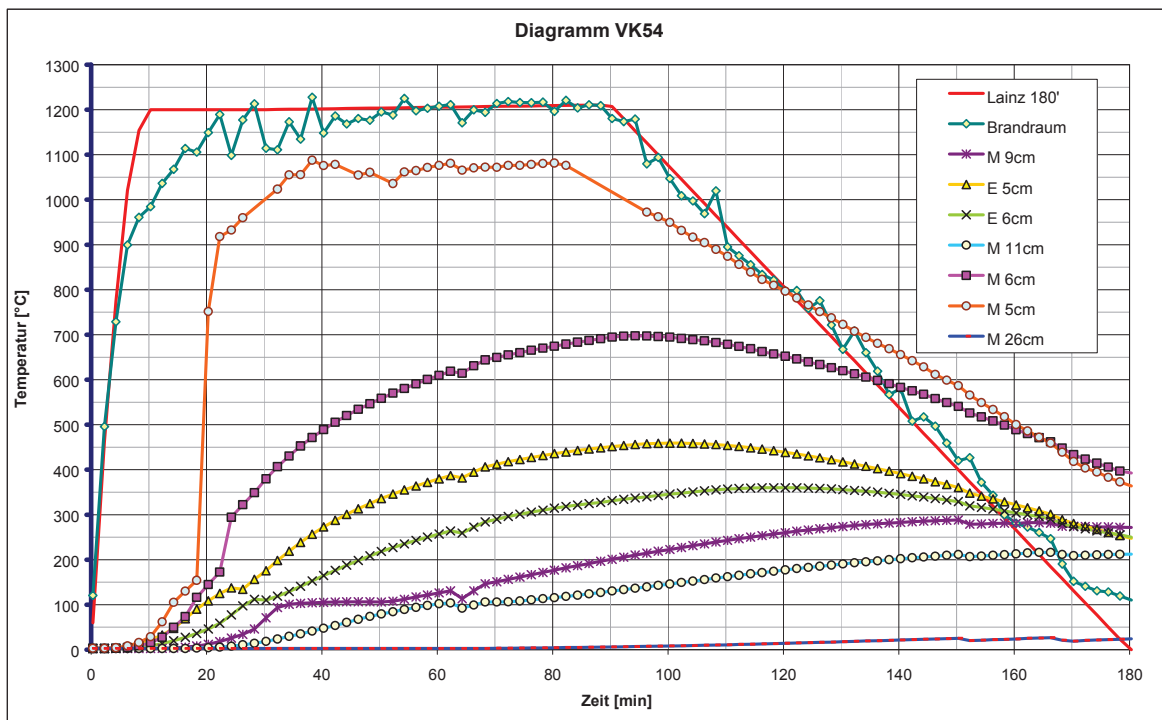
Abb. 39: Sondentemperaturen VK54
