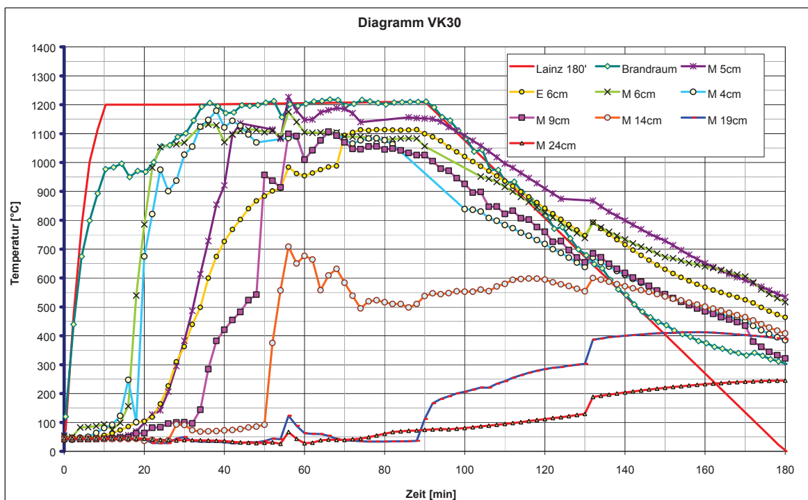
Abb. 28: Sondentemperaturen VK30
