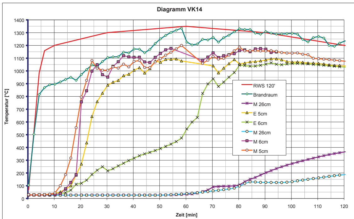
Abb. 14: Sondentemperaturen VK14
