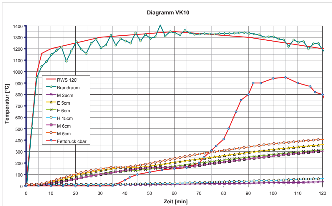
Abb. 10: Sondentemperaturen VK10
