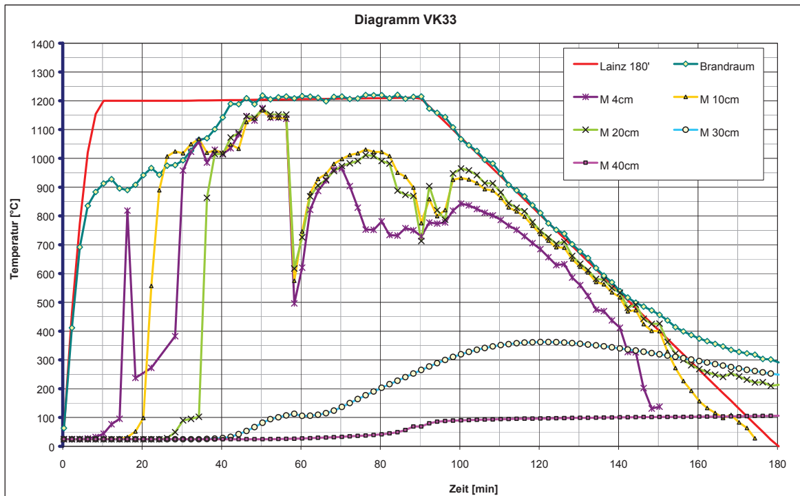
Abb. 31: Sondentemperaturen VK33
