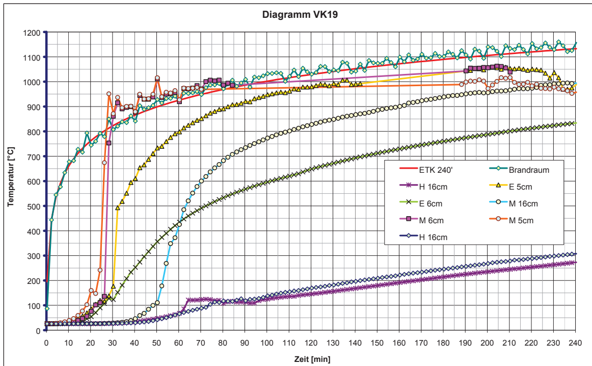
Abb. 19: Sondentemperaturen VK19
